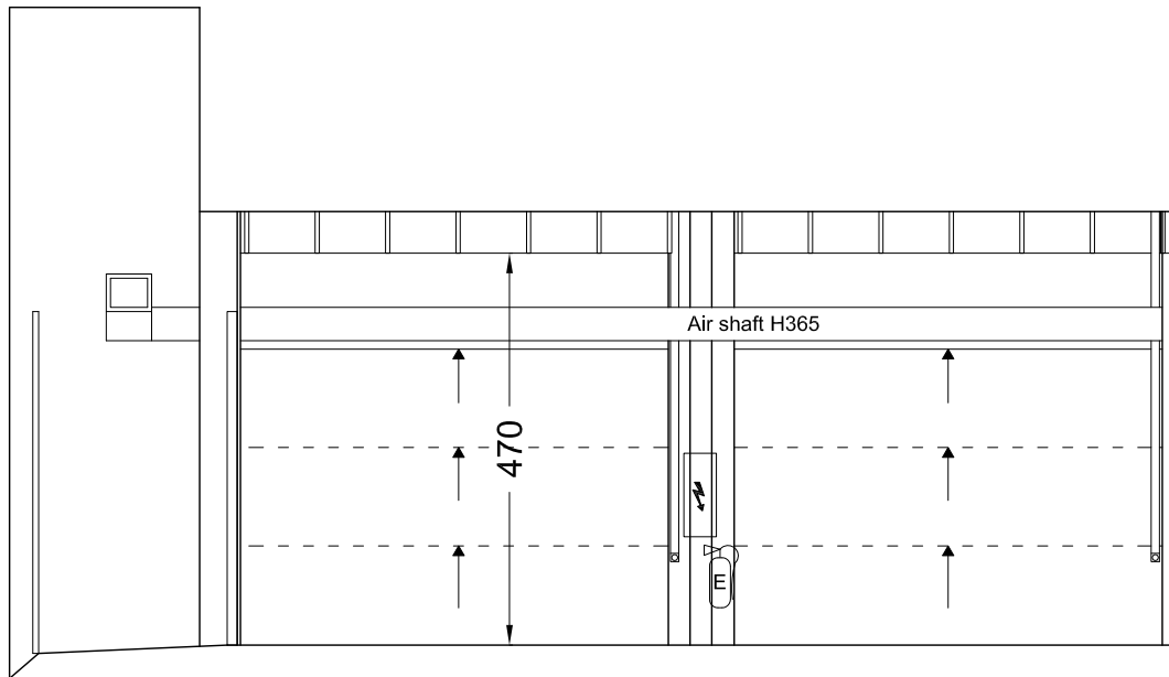
Sezione AA'
