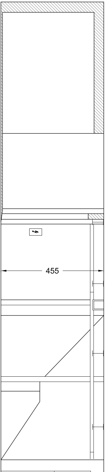
Sezione AA'
